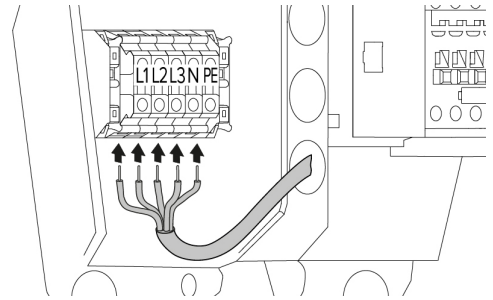
Fig. 9 : raccordement de l'alimentation électrique (exemple : fonctionnement triphasé)
