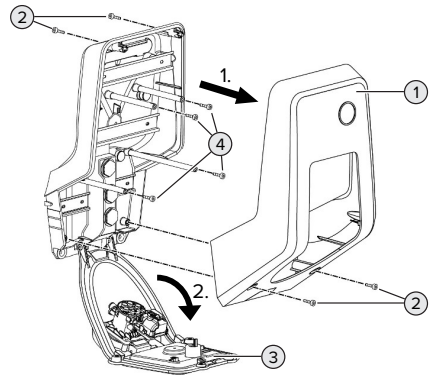
Kuva 6: Tuotteen avaaminen
