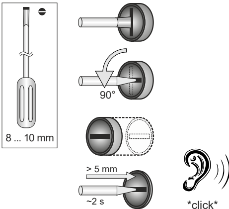
Abb. 21: Fehlerstromschutzschalter prüfen
