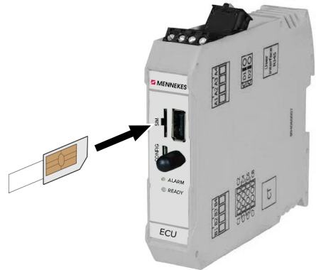
Abb. 13: SIM-Karte einsetzen
