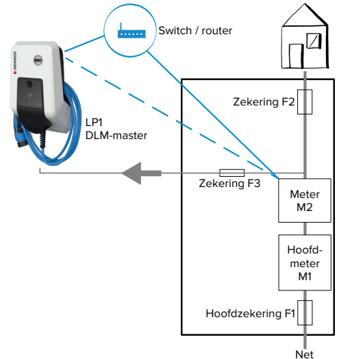
Afb. 16: Energiesmeter meet externe verbruikers en laadstations (totaalverbruik)
