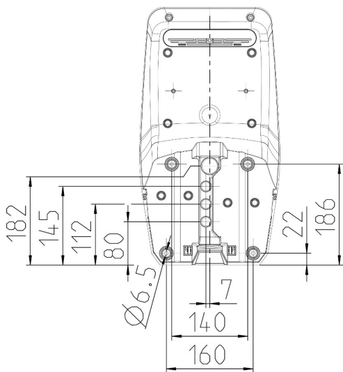
Fig. 7: Boredimensjoner [mm]
