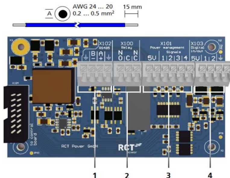
Obr. 6-1 Deska vstupů/výstupů
