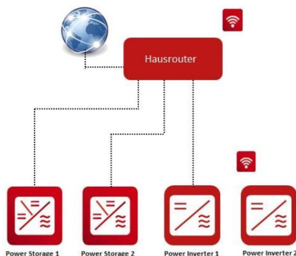
Obrázek 2: Zasíťování zařízení přes router [zde 4 účastníci]
