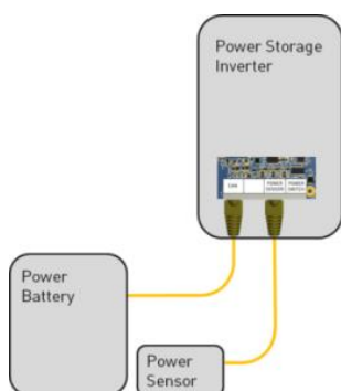
Doplňková komunikace se jednotkou Power Sensor
