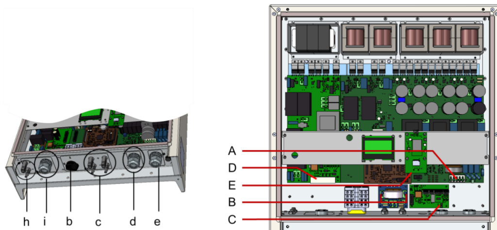
Obr. 5-1 Přehled konektorového oddílu a vnitřních propojovacích prvků
