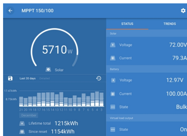
Snímek obrazovky aplikace VictronConnect zobrazující data v reálném čase a historická data.
