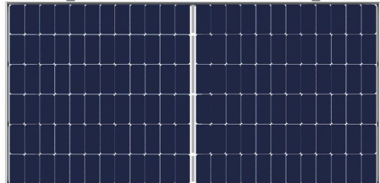
Instalace pomocí šroubů do 4 vnějších otvorů (nosník je kolmo k podélným stranám)
