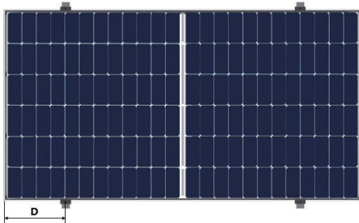
Instalace rámového modulu s úchytkami na podélných stranách (nosník je kolmo k podélným stranám) (délka svorky \geq 40 mm)
